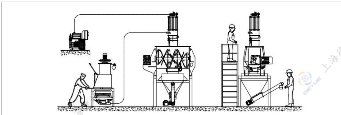
配置 A：人工投料站投料→气力输送机输送→混合→成品料仓→螺旋出料→人工包装
