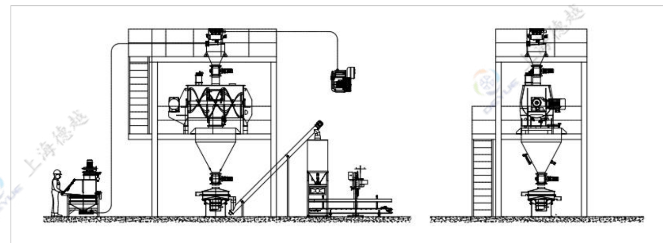
配置 B：人工投料站投料→混合→动态料仓→螺旋出料→包装机包装
