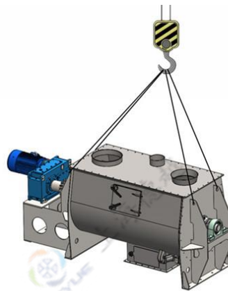
图 6.2 设备吊装示意图
