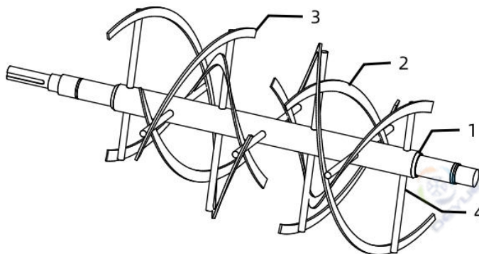
【图 4.2-1】搅拌器结构
