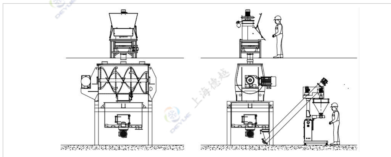
配置 B：人工投料站投料→混合→动态料仓→螺旋出料→包装机包装
